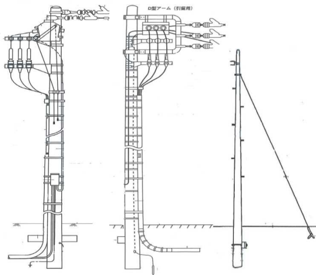
例) マルヒ装柱 例) Dアーム装柱 例) 低圧引込・支線
